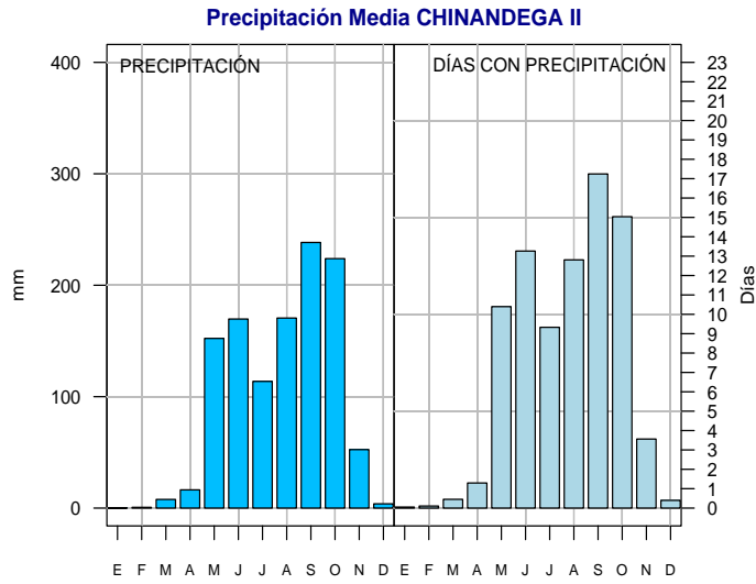
Figura 8. Climograma de precipitación En Chinandega II.
