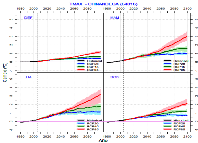
Figura 9. Incrementos de temperatura máxima.
